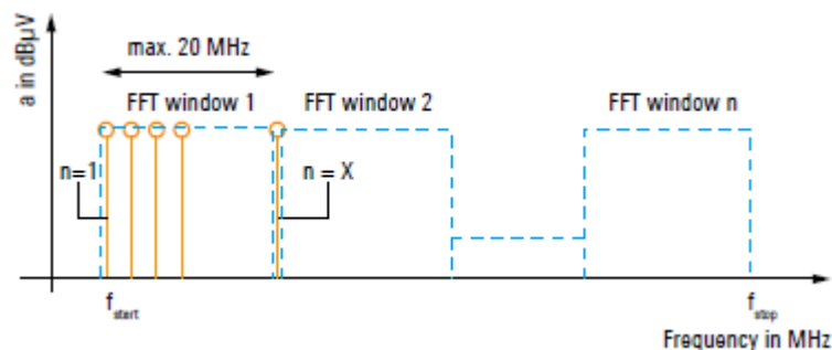
Рис. 1-17. Механизм обработки сигналов в режиме панорамного сканирования
