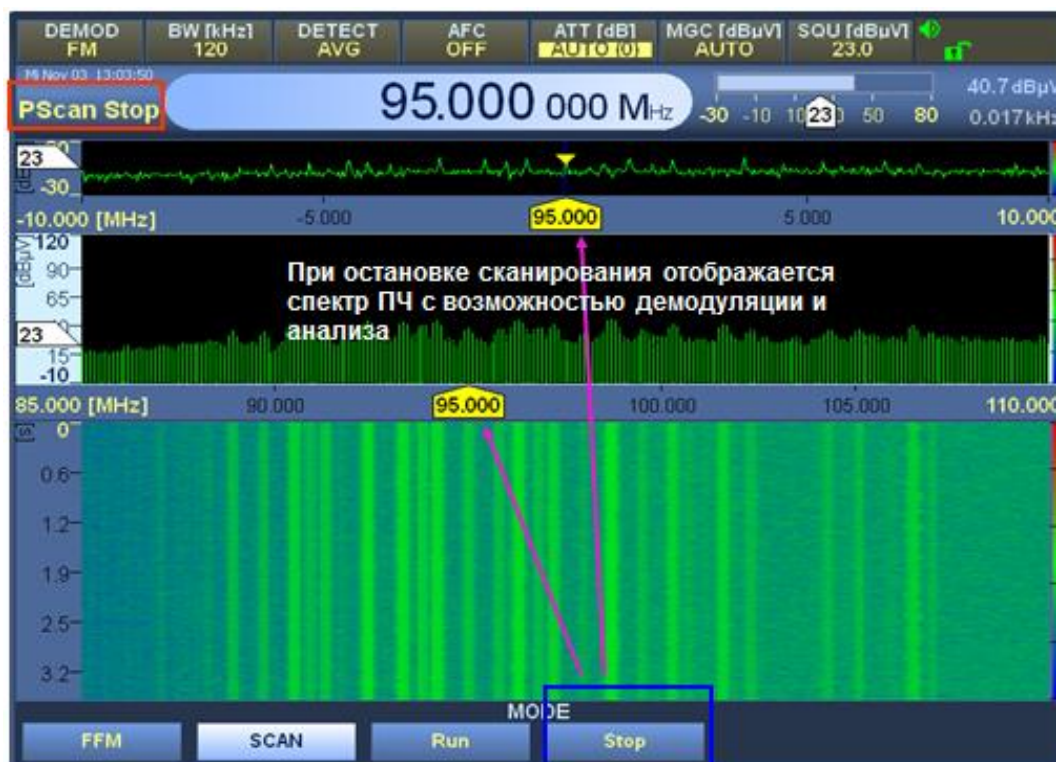
Рис. 1-2. R&S®EB500. Режим панорамного сканирования
