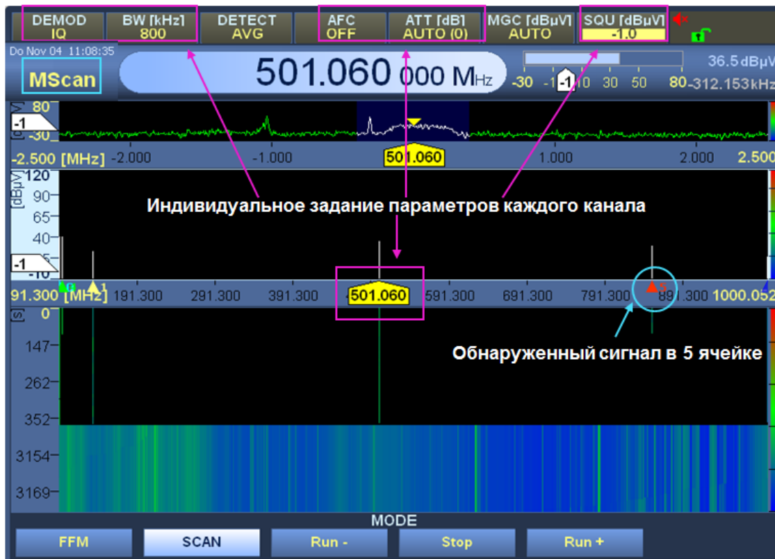
Рис. 1-6. R&amp;S®EB500. Функция сканирования по памяти
