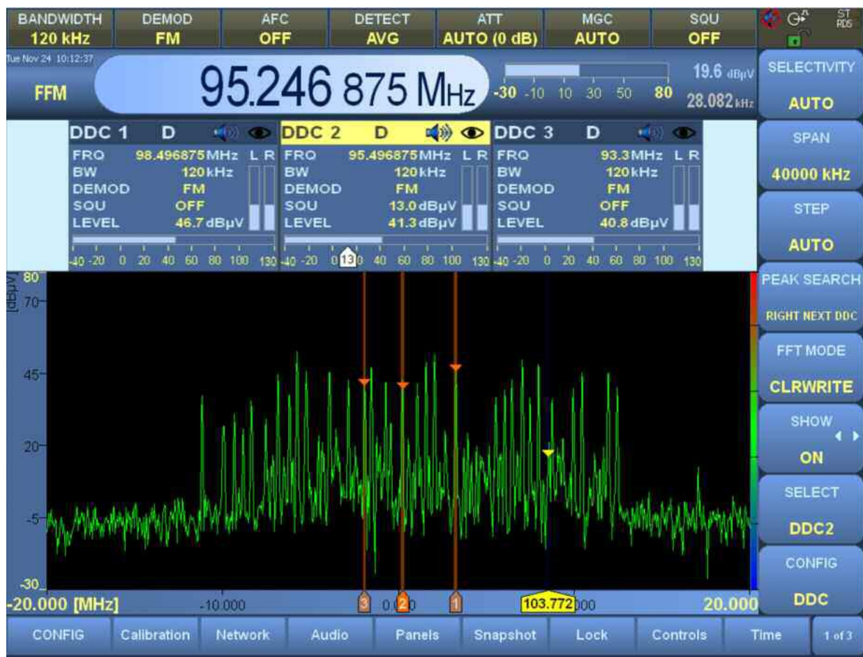
Рис. 1-3. Опция цифровых приемников R&S®EB500-DDC
